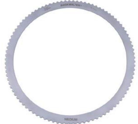
70-113 Küçük Ø 215 mm 70-114 Orta Ø 265 mm 70-115 Büyük Ø 315 mm Yuvarlak çember
