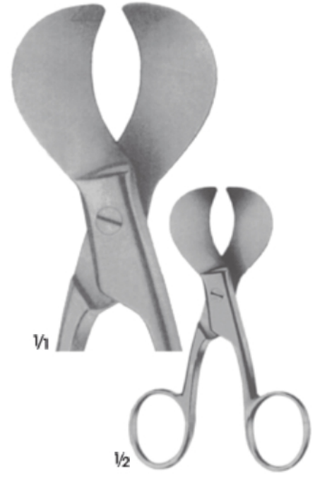
42-598 Göbek kordonu makası Umbilical cord scissors 10.5 cm
