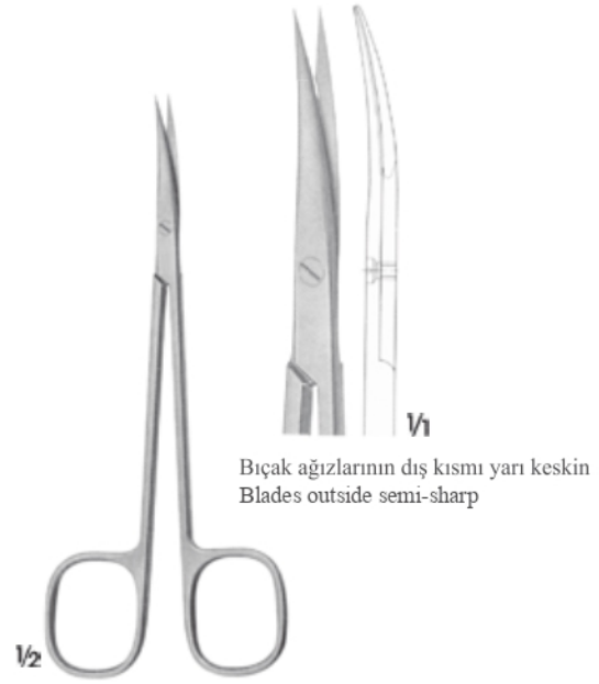
42-361 Diseksiyon, sinir makası Nerve dissecting scissors 14 cm
